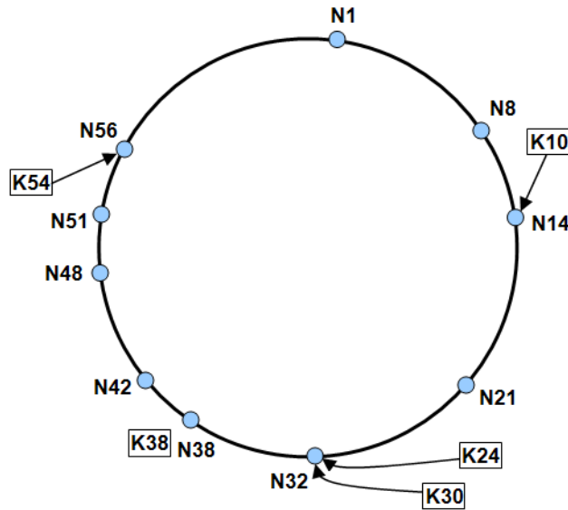
FIG. 2.9 – Répartition des clés
