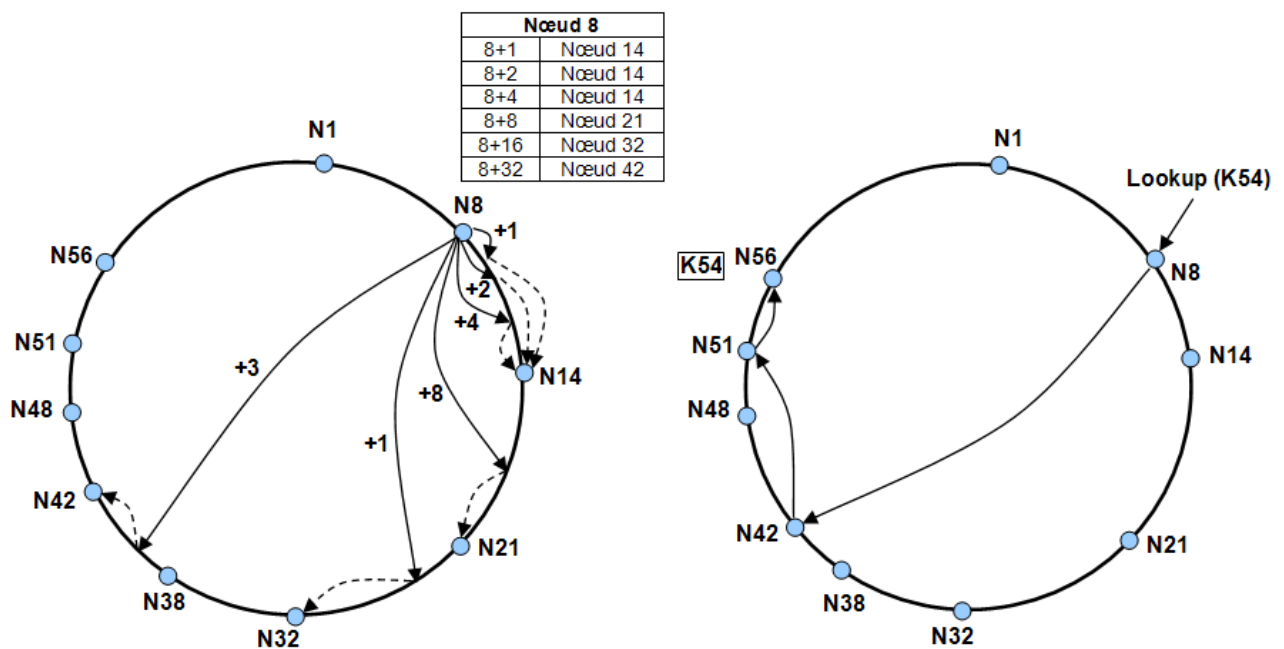
FIG. 2.11 – Répartition des clés
