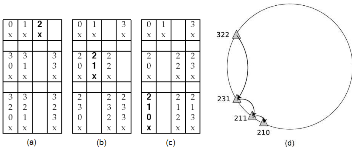
FIG. 2.6 – Exemple de routage par préfixe dans Pastry (simplifié). (a) Table de routage du noeud 322, (b) Table de routage du noeud 231, (c) Table de routage du noeud 211, (d) Chemin du message.
